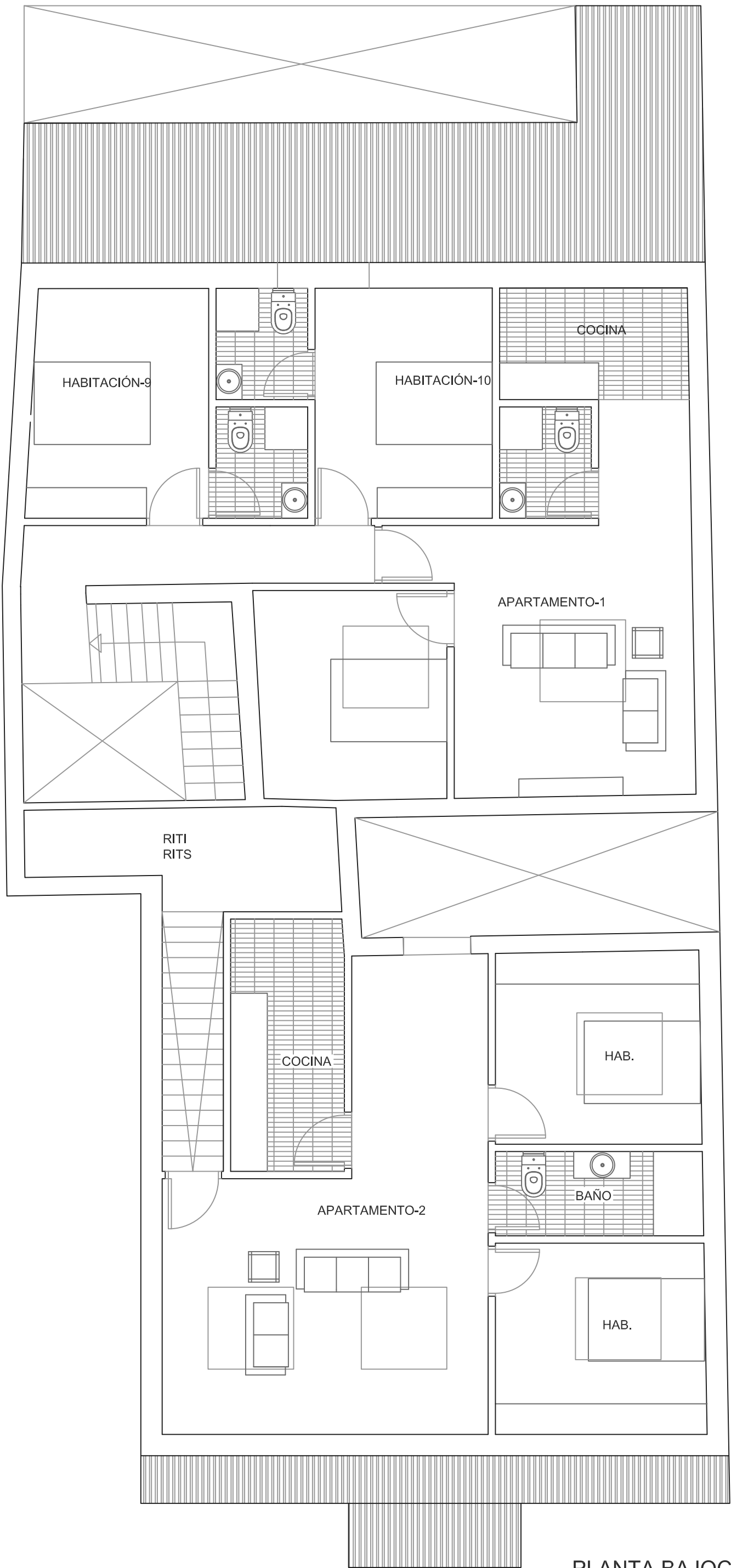
PLANTA BAJOCUBIERTA
